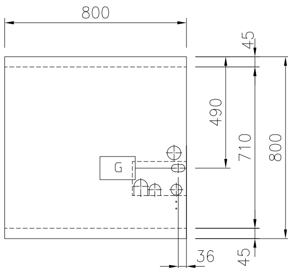
Boven aanzicht
