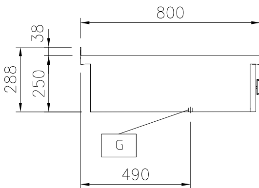
Zij aanzicht
